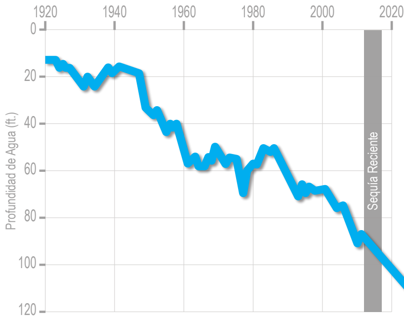
Profundidad Promedia de Agua Subterránea - Distrito de Irrigación de Fresno
